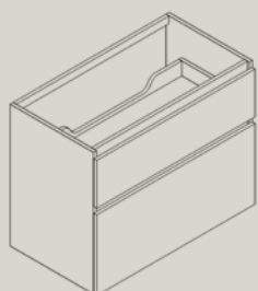
Maatvoering (B x D x H) 1000x460x650 mm
